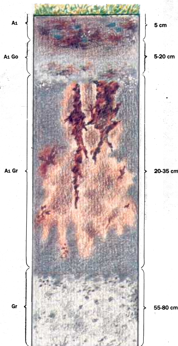
Fig. 7. Perfil de un suelo de manglar (Typic sulfaquent; Thionic fluvisol; suelo salino con sulfato-reducción) según Duchafour, 1977.
