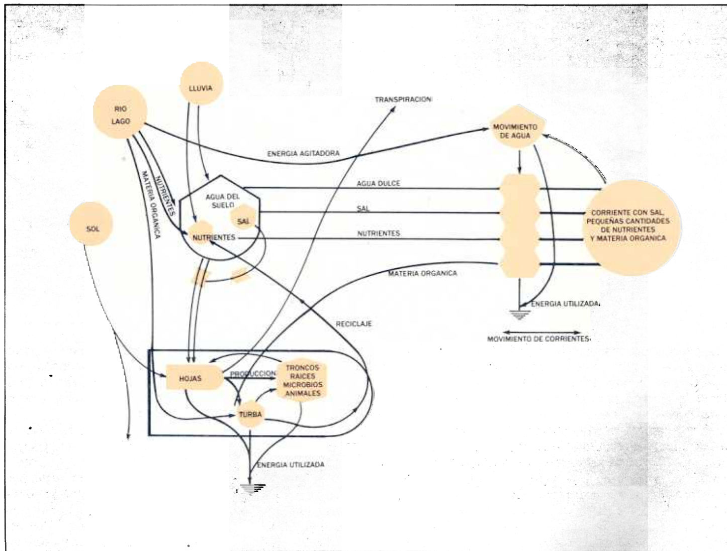
Fig. 11. Modelo del flujo energético de ecosistemas de manglares. Los símbolos de Odum (1971). El modelo representa acumulaciones de biomasa, los procesos de productividad, respiración y reciclaje; el ingreso y salida de nutrientes (ingreso neto) y materia orgánica (salida neta); y los factores (tanto internos como externos) que se cree que controlan estas tasas. Cintron et al. (1978).
