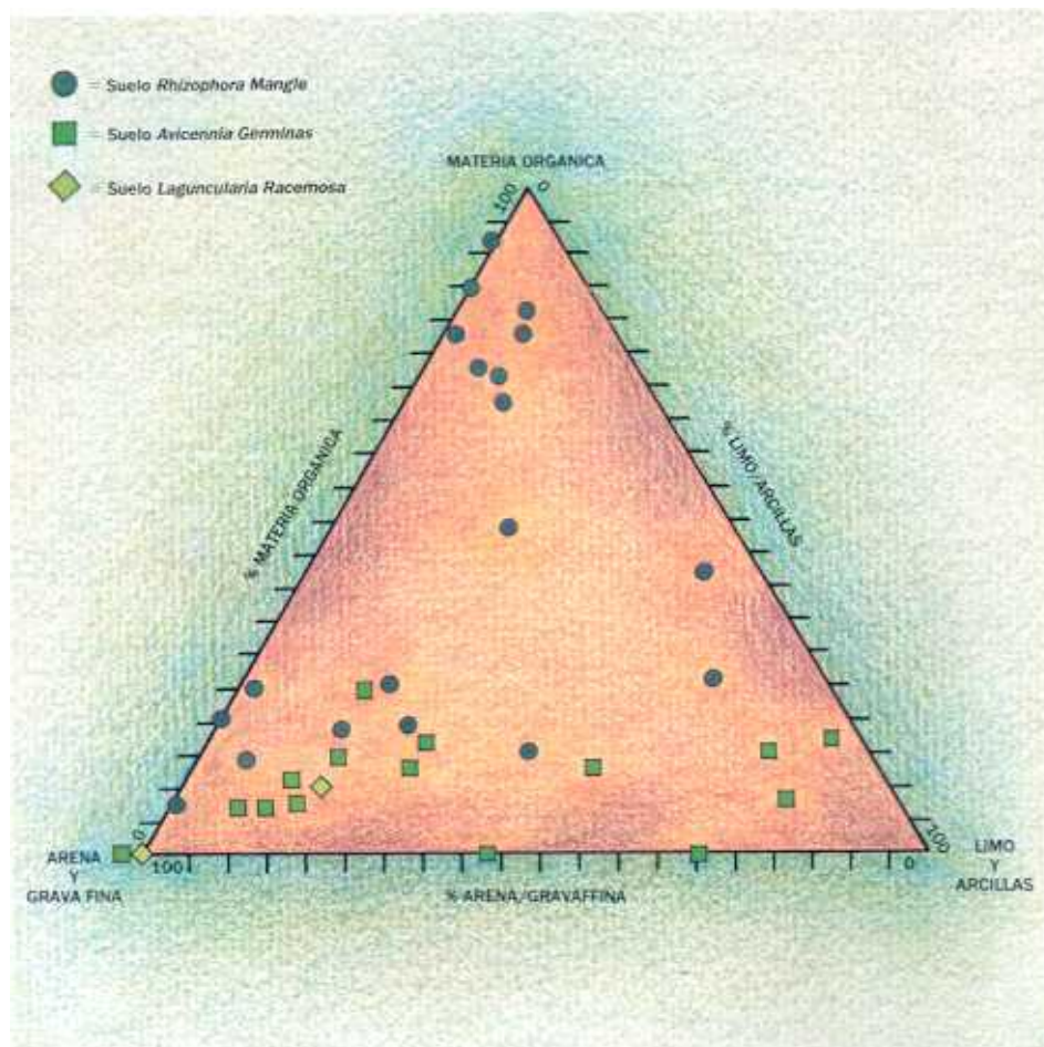
Fig. 6. Triángulo granulométrico indicativo de la composición de distintos suelos del manglar
