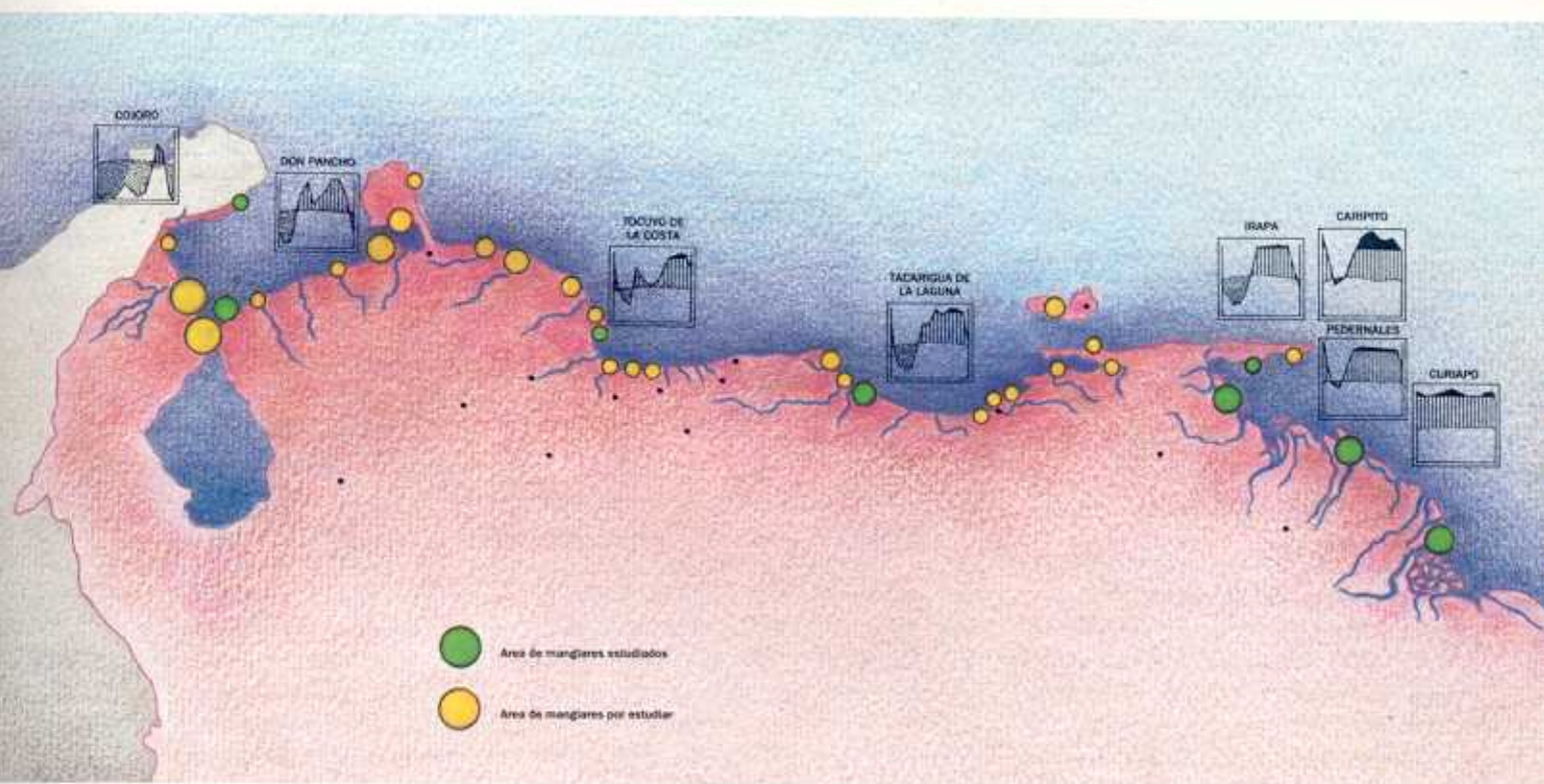
Fig. 12. Gradiente climático de la costa venezolana poblada por manglares (ver círculos) indicada por la representación gráfica climática de Climadiagramas (explicación en el texto)
